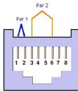
10BaseT (802.3) „
